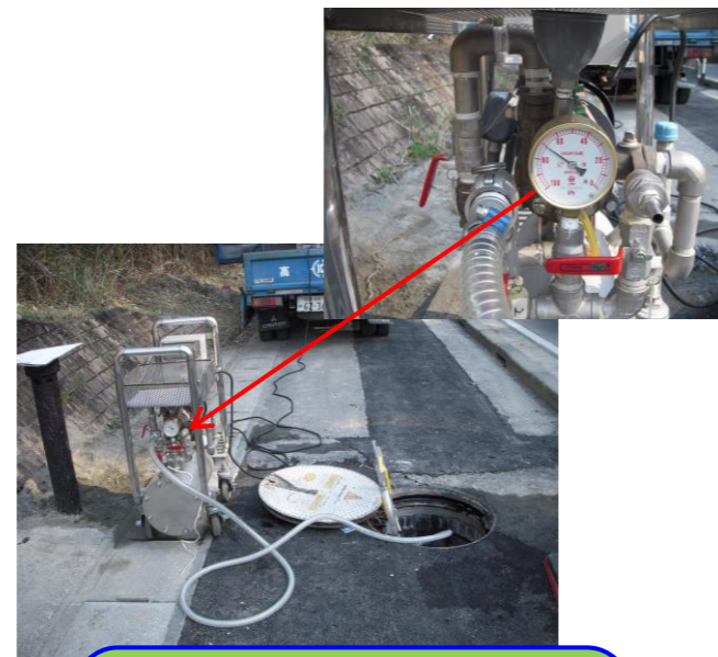
気密試験 管路内に負圧(70KPA)をかけて1時間保持し、接続不良箇所がないか確認をします。
